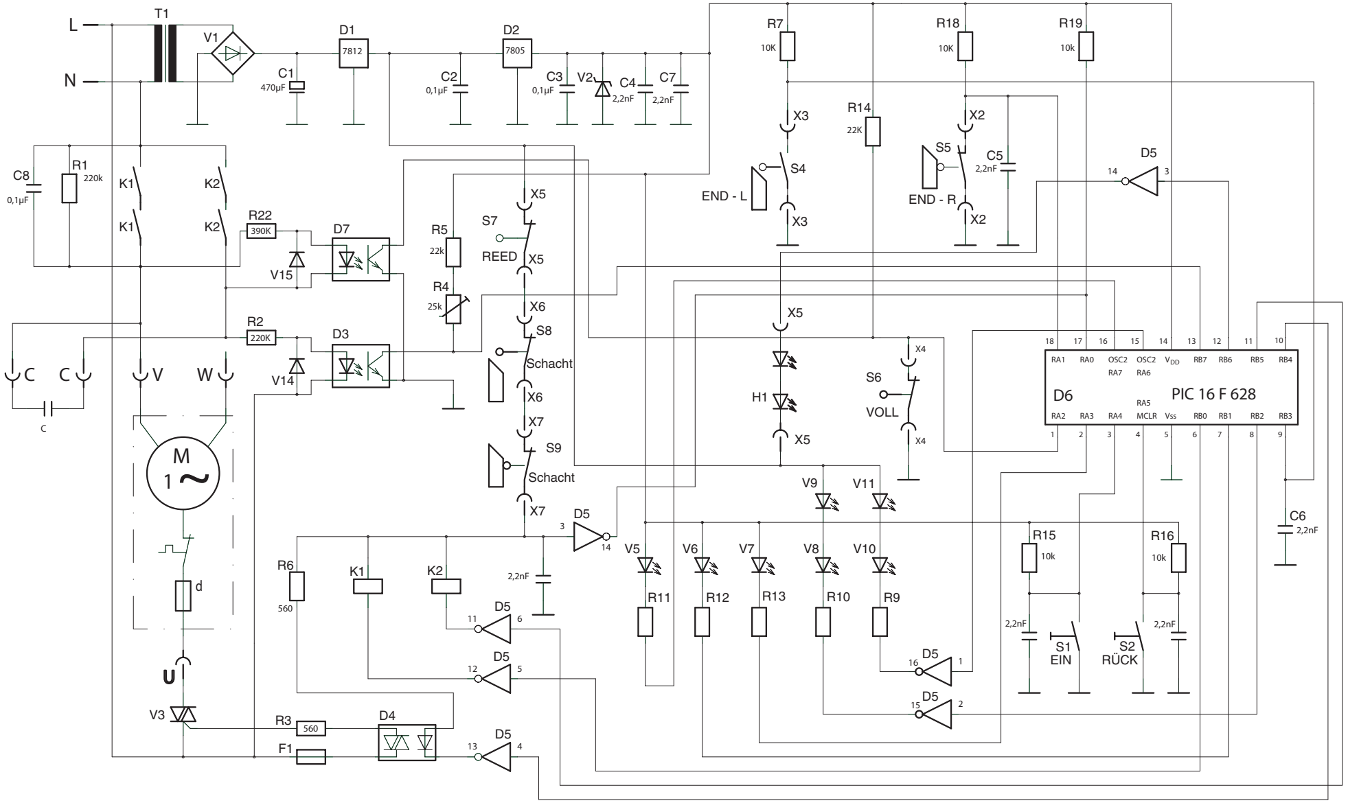
Stromlaufplan 0101HDP A Schema de circuit électrique 0101HDP A Wiring diagram 0101HDP A
