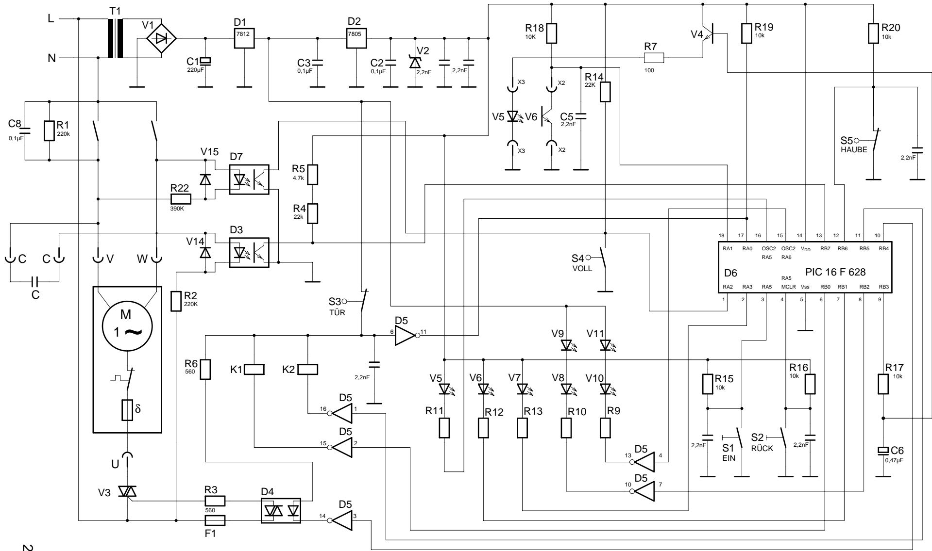
Stromlaufplan 2360 A schema de circuit électrique 2360 A wiring diagram 2360 A
