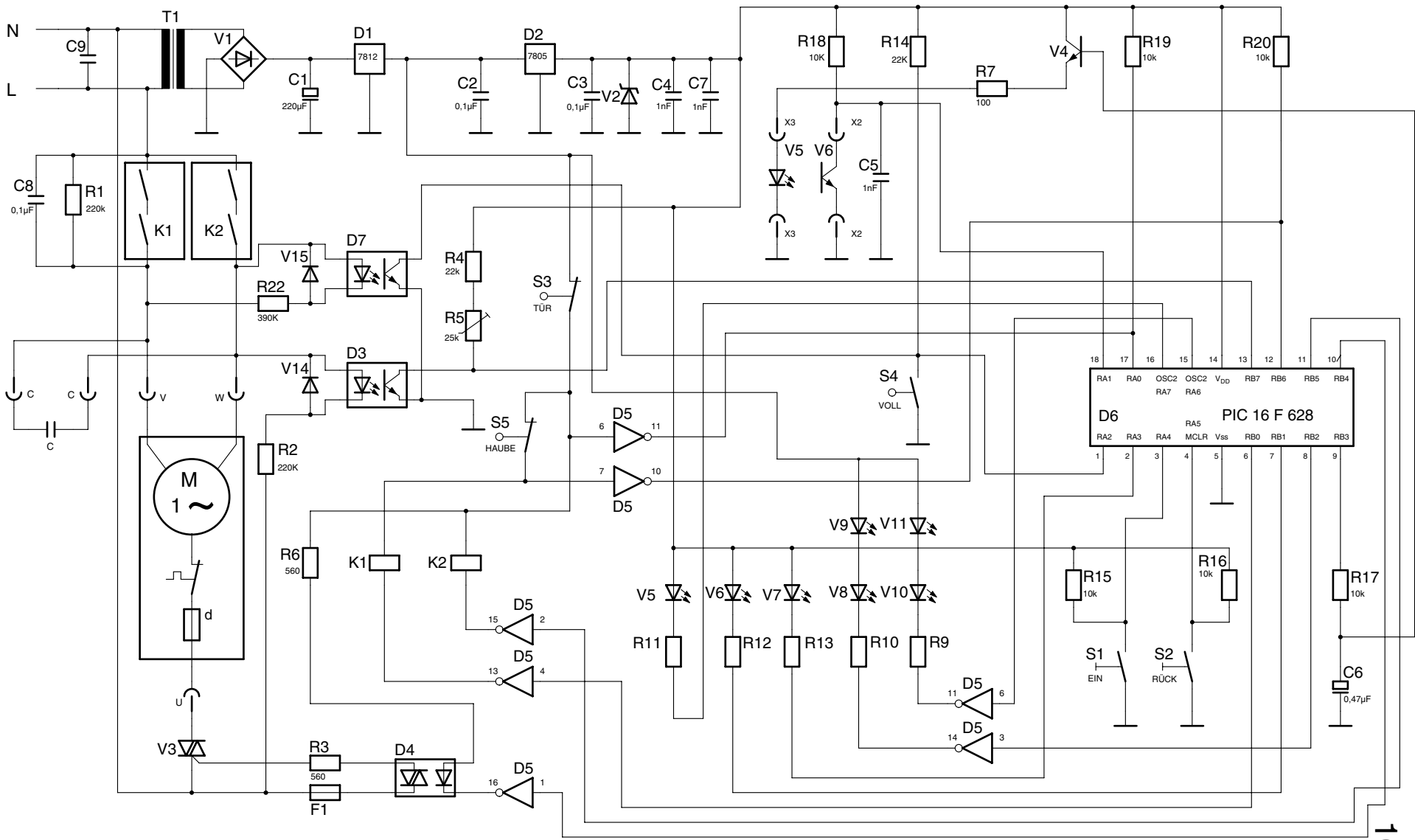
Stromlaufplan 2503 B schema de circuit électrique 2503 B wiring diagram 2503 B
