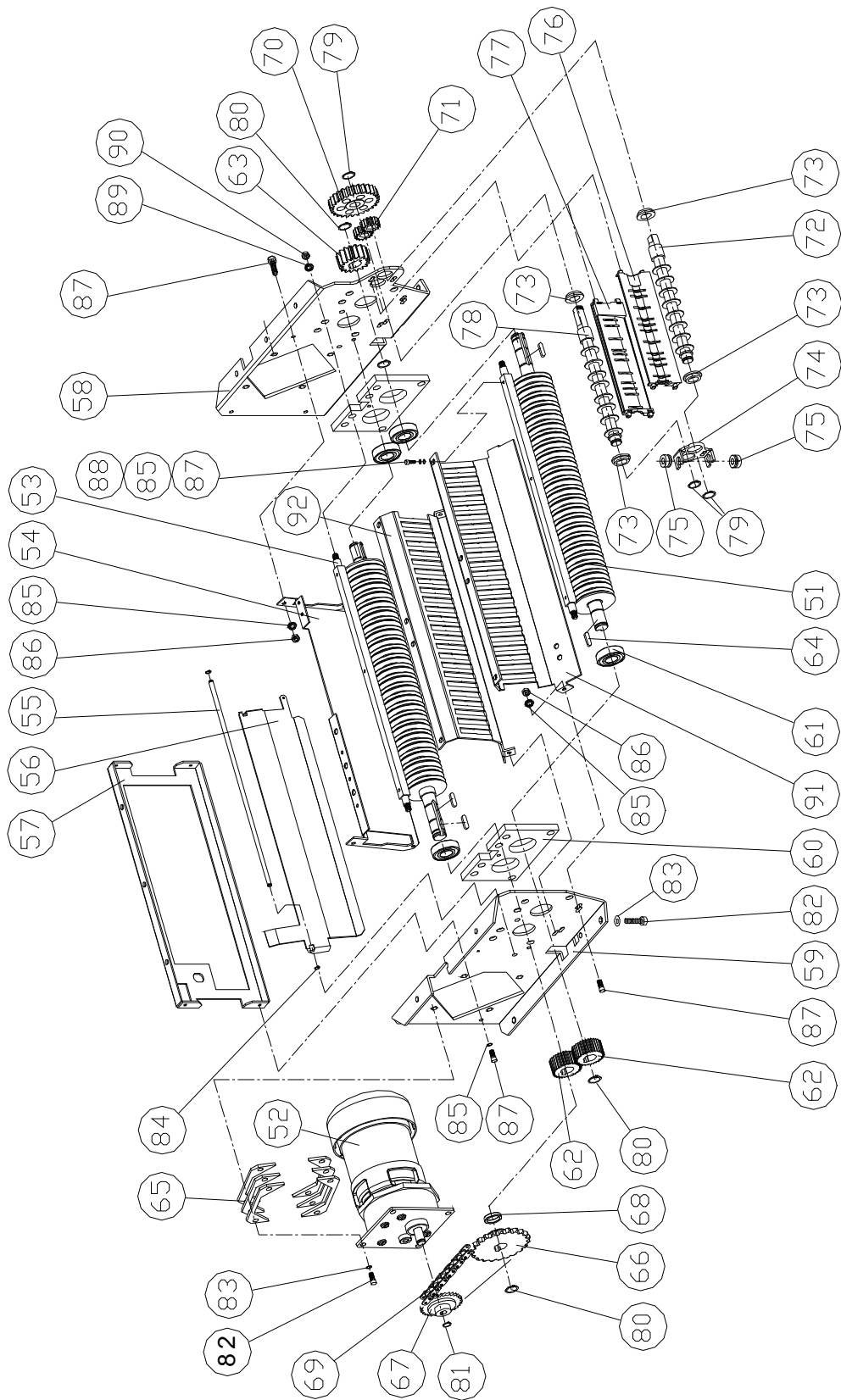
DISEGNO 3A /DRAWING 3A
