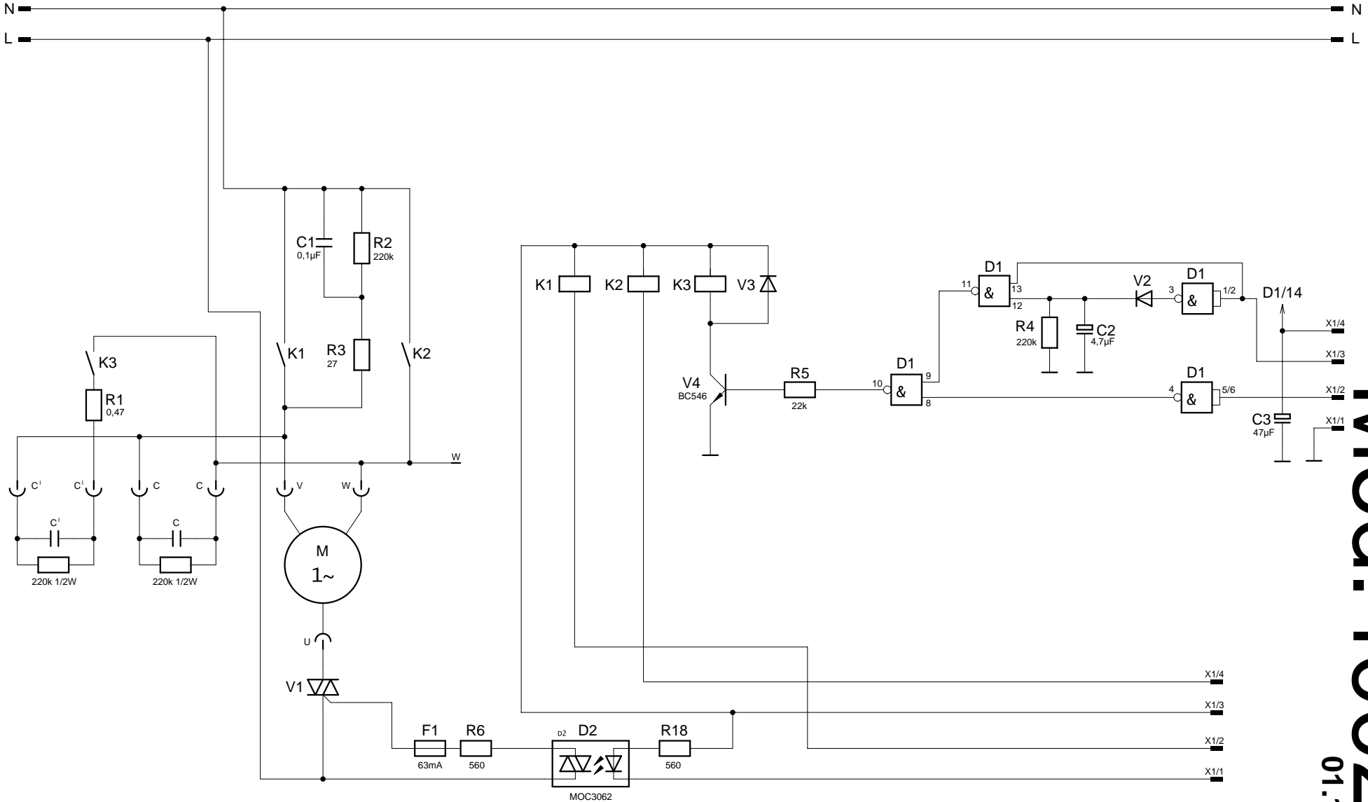
Stromlaufplan 4002 B schema de circuit électrique 4002 B wiring diagram 4002 B
