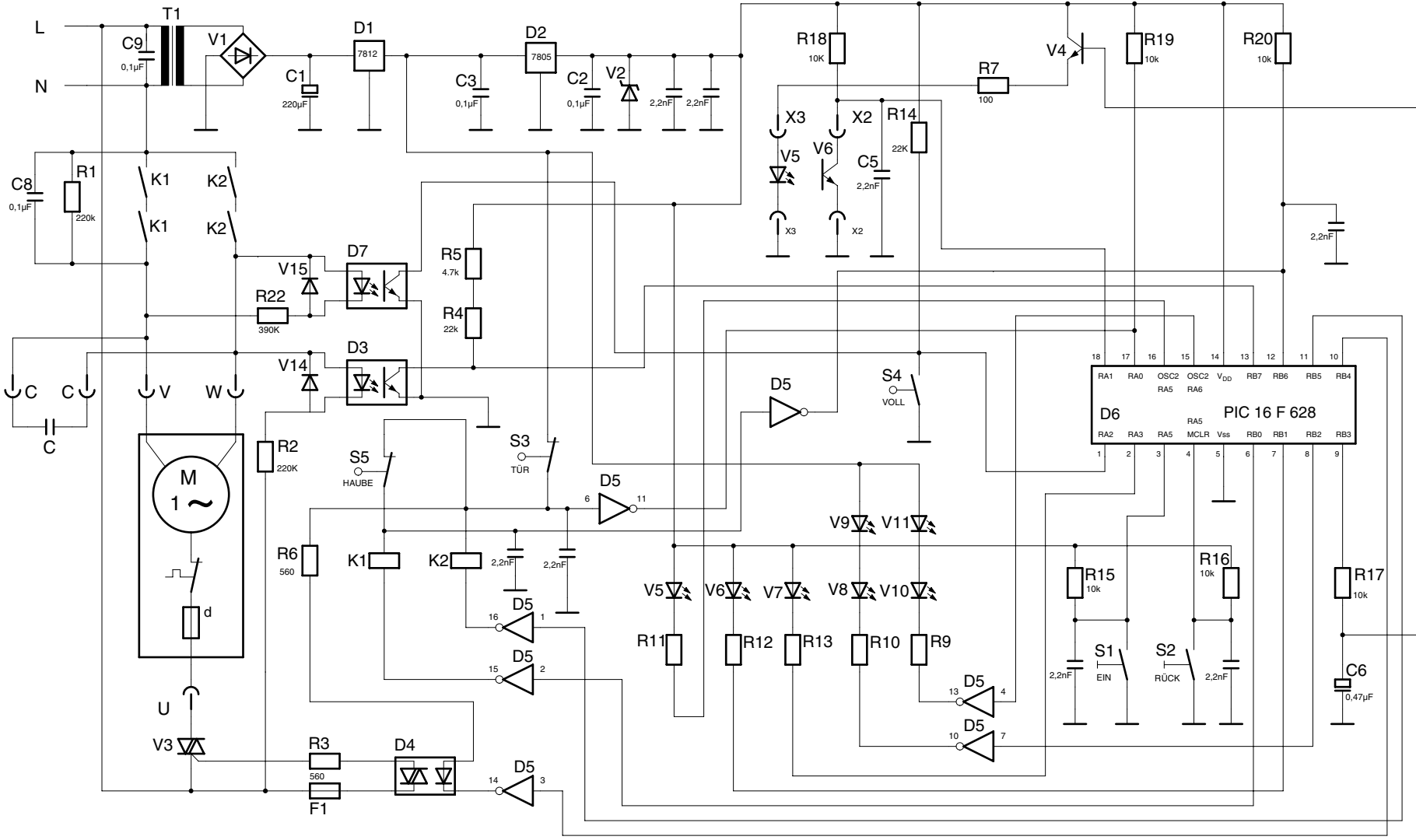
Stromlaufplan 2404 B schema de circuit électrique 2404 B wiring diagram 2404 B
