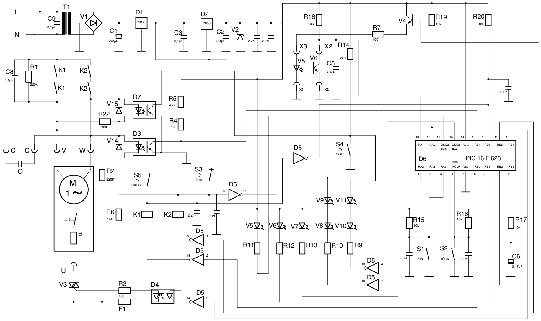
Stromlaufplan 2360 B schema de circuit electrique 2360 B wiring diagram 2360 B
